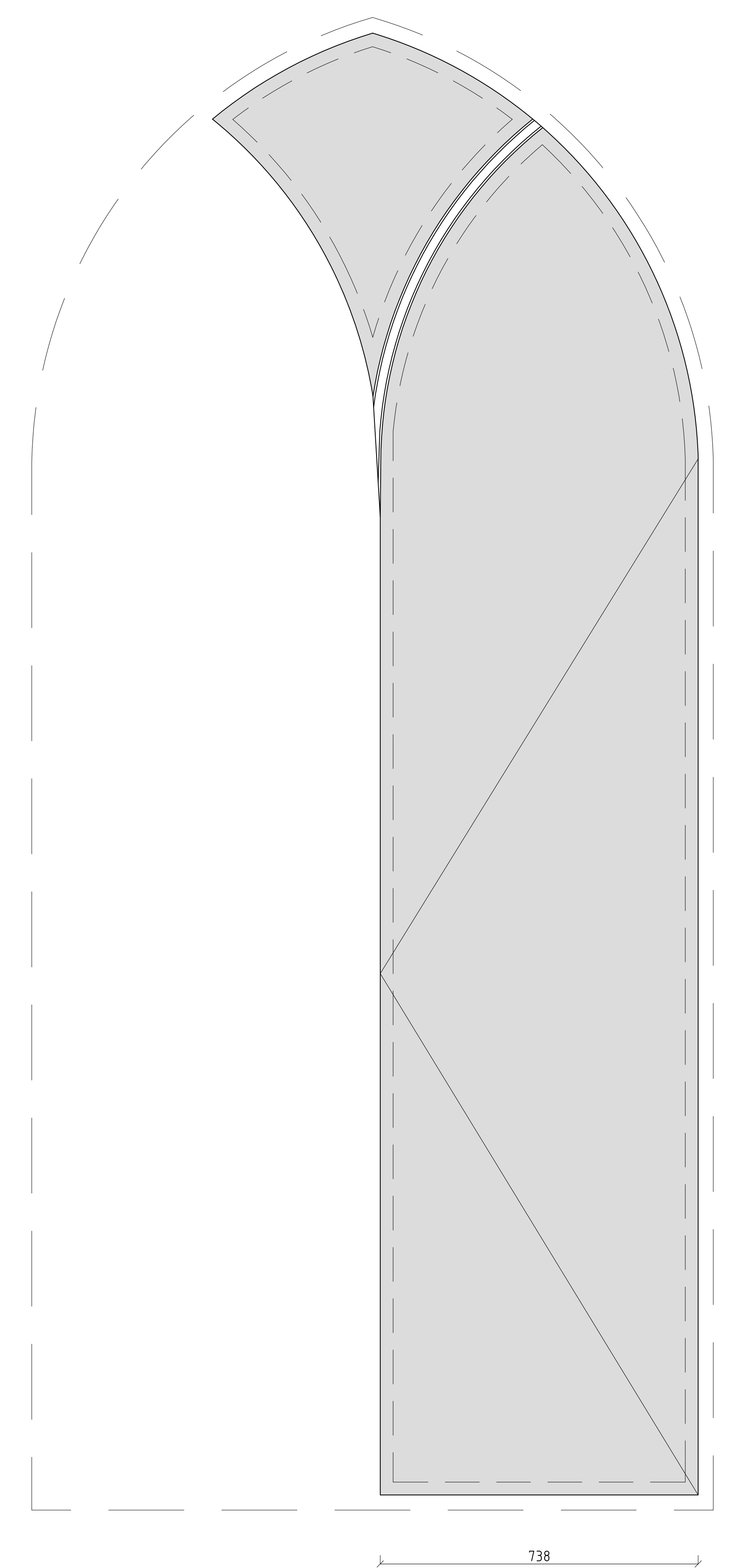
AANZICHT DRAAIEND DEEL RECHTS
